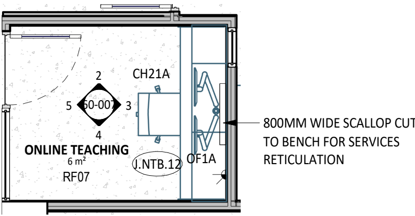
1 PLAN DETAIL 30-01 1 : 50
